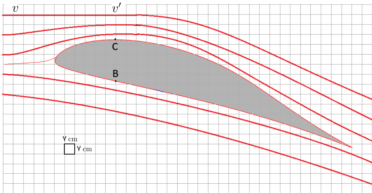
شکل ۱: هوابرد (مقطع بال هواپیما)، در این شکل طول هر ضلع مربع ۱ cm است.
